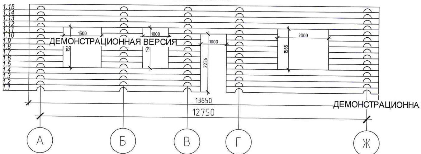
РАЗВЕРТКА ПО ОСИ 1
